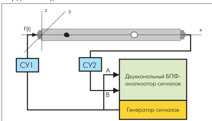
Блок-схема установки для исследования структуры и физических свойств материалов: СИ1 и СИ2 – входной и выходной согласующие усилители
