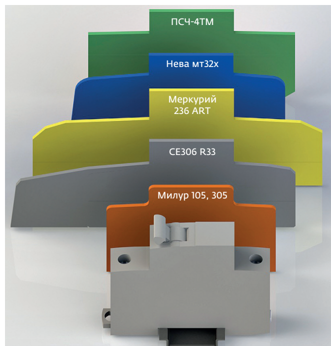
Рис.4. Габариты различных счетчиков по ширине
