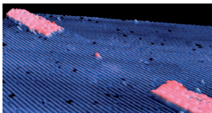
Рис.1. Изображение одноатомного "транзистора": на поверхности кремния внедренные атомы фосфора. Изображение получено на сканирующем туннельном микроскопе (СТМ)
