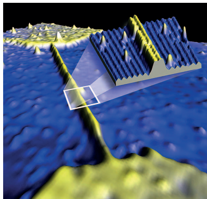
Рис.4. СТМ-изображение кремний-фосфорного проводника
