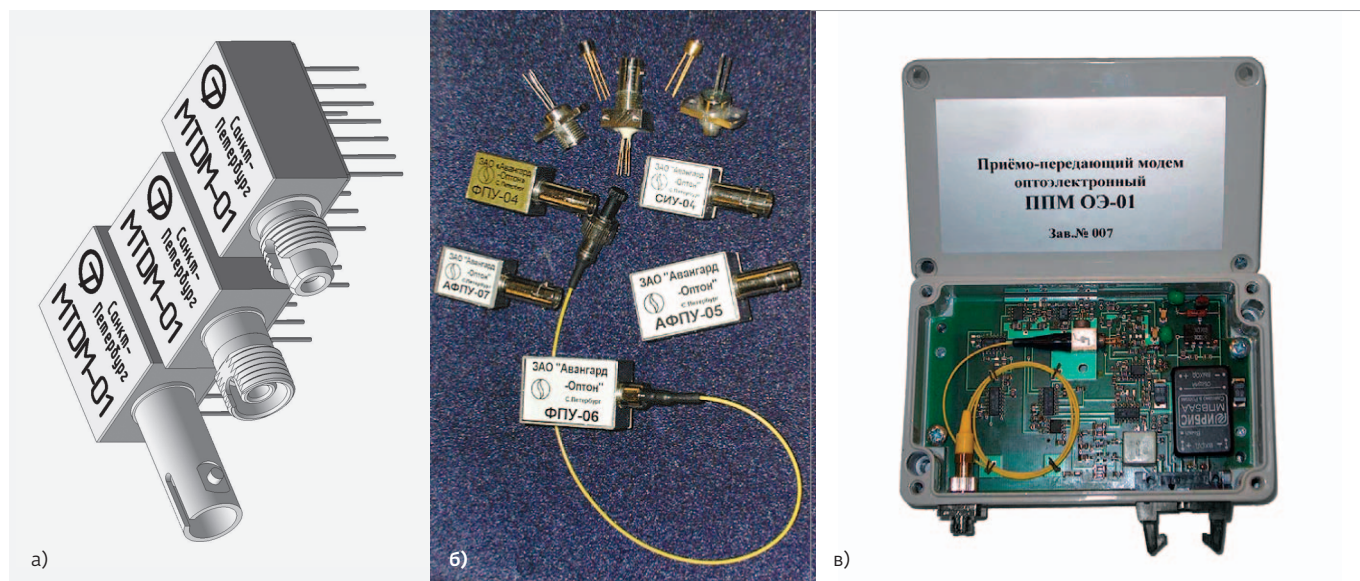
Рис.5. Светоизлучающие (а) и фотоприемные (б) оптоэлектронные модули и приемо-передающий модем (в)
