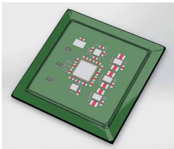
Рис.1. Модель многокристальной сборки на основе DSP-процессора 1967ВЦ2Т
