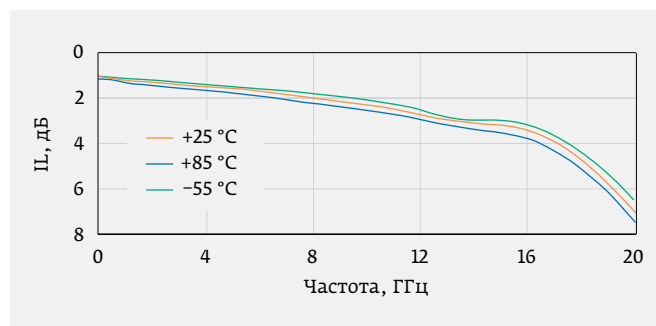
Рис. 16. Зависимости вносимых потерь от частоты в поглощающем переключателе НМС-С058 (Analog Devices) при различных значениях температуры окружающей среды
