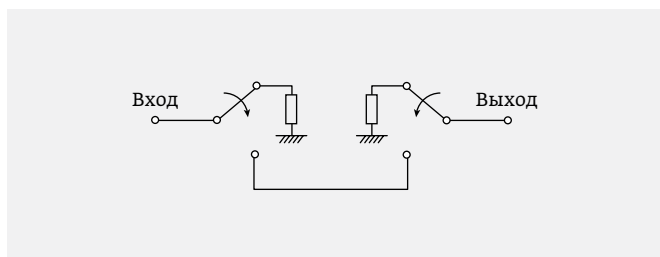
Рис. 10. Схематичное изображение структуры переключателей НМС-С019 и НМС-С583 (компания Analog Devices)
