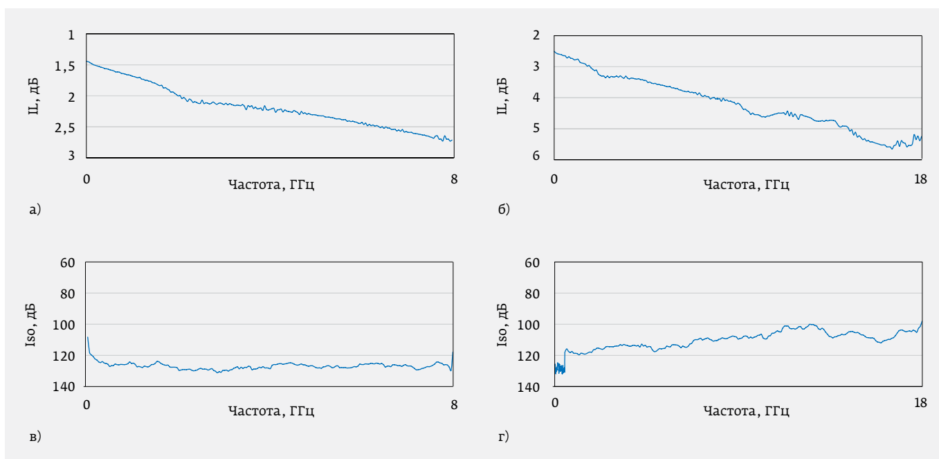
Рис. 17. Зависимости вносимых потерь (а, б) и развязки (в, г) от частоты для SPDT-переключателей U9397A (а, в) и U9397C (б, г), выпускаемых компанией Keysight
