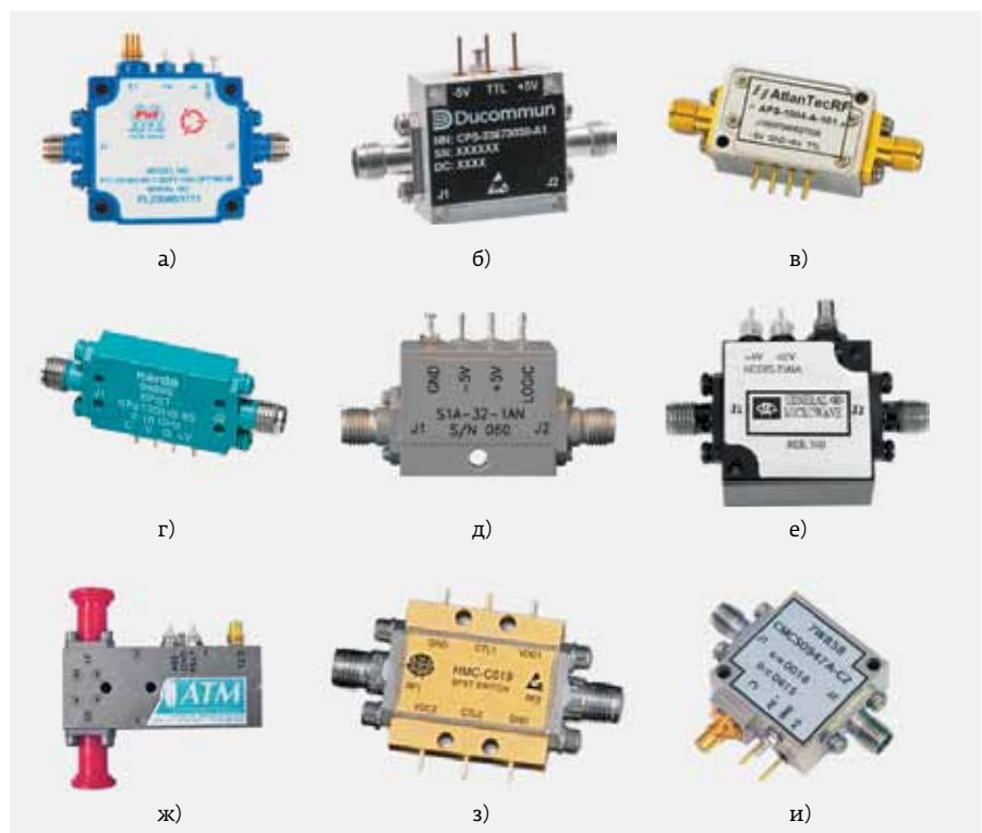
Рис. 6. Конструкции модульных SPST-переключателей: а – PIT-DC40C-65-T-292FF-1NS (PMI); б – CPS-33673030-A1 (Ducommun Technologies); в – APS-1004-A-101 (AtlantecRF); г – SP213DHS-80 (Narda Microwave); д – S1A-32-1AN (Mercury Systems); е – F192A (Kratos); ж – S1517D (ATM); з – HMC-C019 (Analog Devices); и – CMCS0947A-C2 (CMC)
