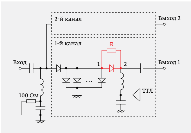
Рис. 12 Принципиальная схема pin-диодного поглощающего SPDT-переключателя (серия SN20-31x, компания CMC)
