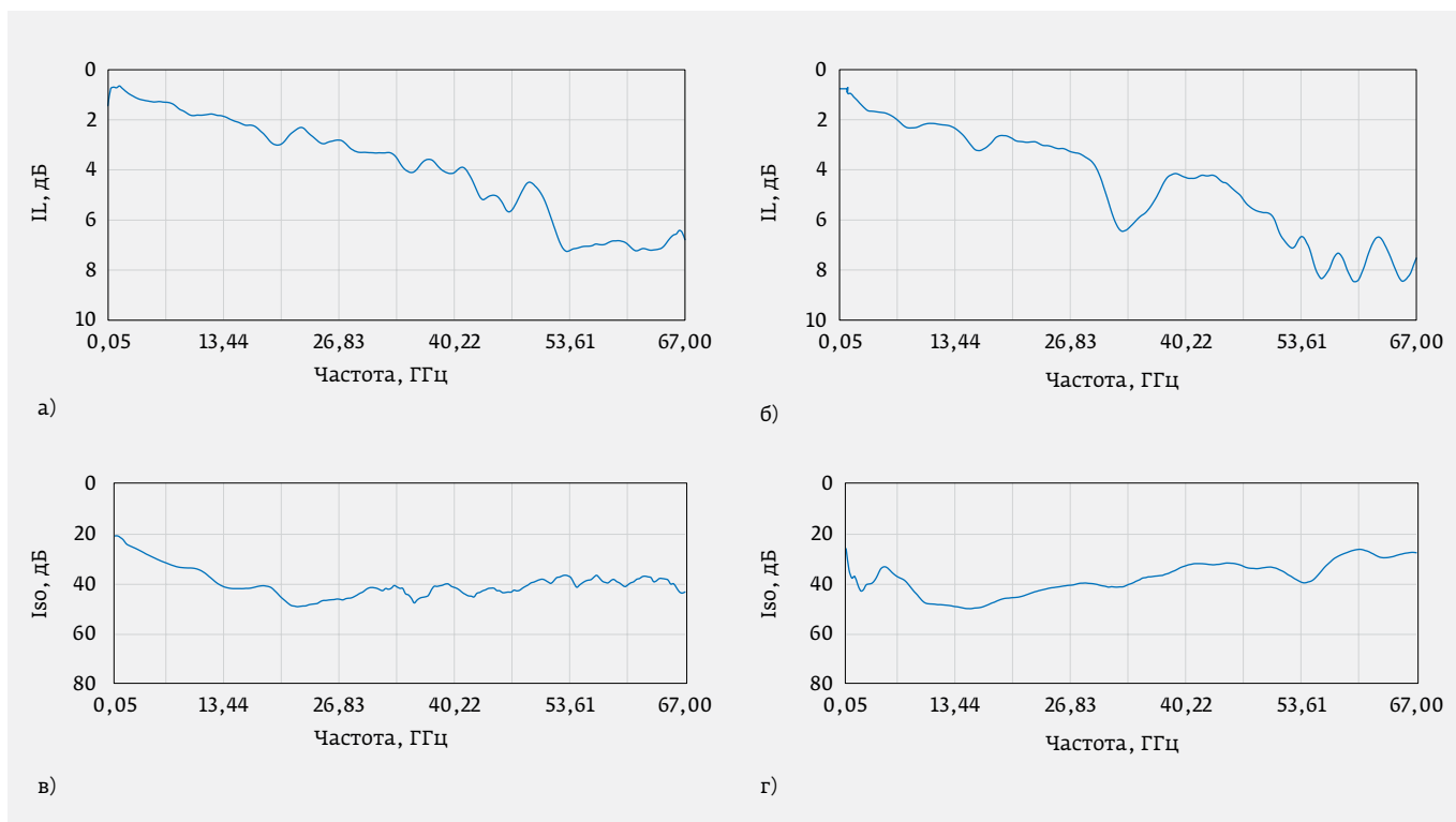
Рис. 9. Зависимости вносимых потерь (а, б) и развязки (в, г) в отражательном PE71S2023 (а, в) и поглощающем PE71S2024 (б, г) переключателях компании Pasternack
