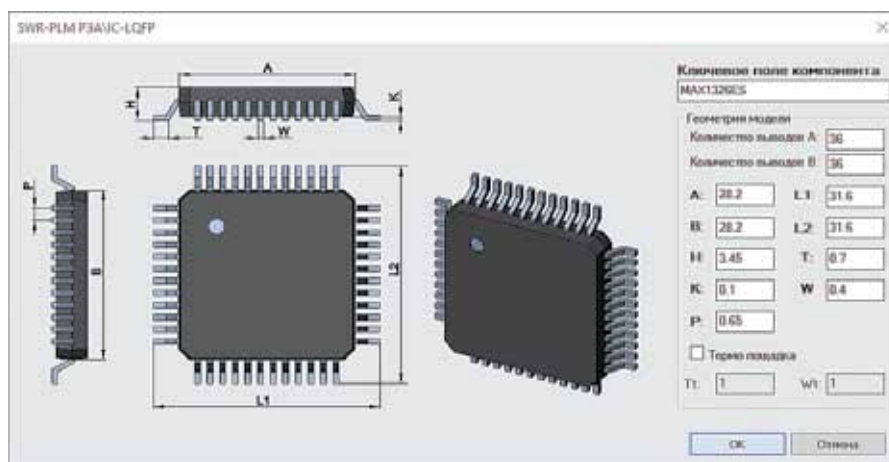
Рис. 3. Библиотечный элемент РЭА
