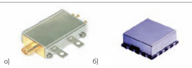
Рис. 2. Управляемые напряжением генераторы ZX95-2500 (а) и ROS-3000V (б)
