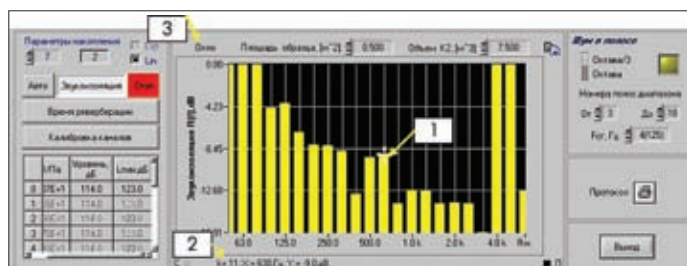
Рис.9. Результаты измерений звукоизоляции образца на модели: 1 – следящий курсор; 2 – поле отображения координат следящего курсора; 3 – элемент управления, задающий тип объекта измерений (окно/дверь)
