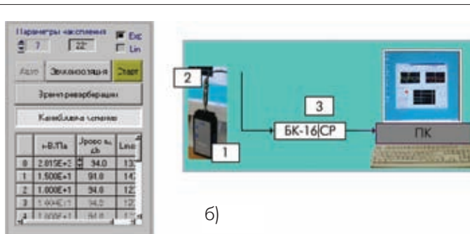
Рис.6. Установки поля управления: а) "режим"; б) блок-схема калибровки измерительного канала: 1 – пистонфон; 2 – измерительный микрофон; 3 – блок коммутации комплекса
