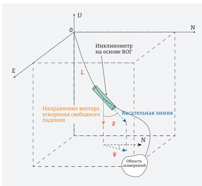
Рис. 1. Параметры скважины [1]
