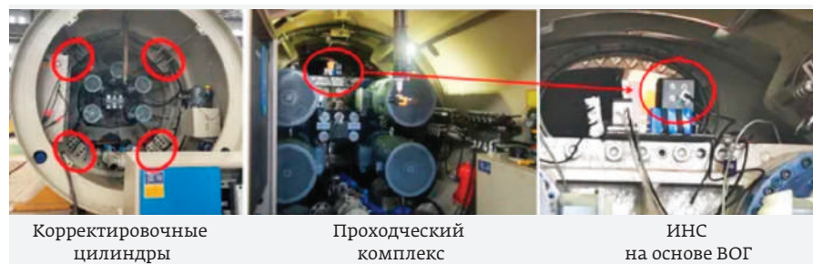
Рис. 6. Модуль на основе ВОГ в машине для микротоннелирования [6]
