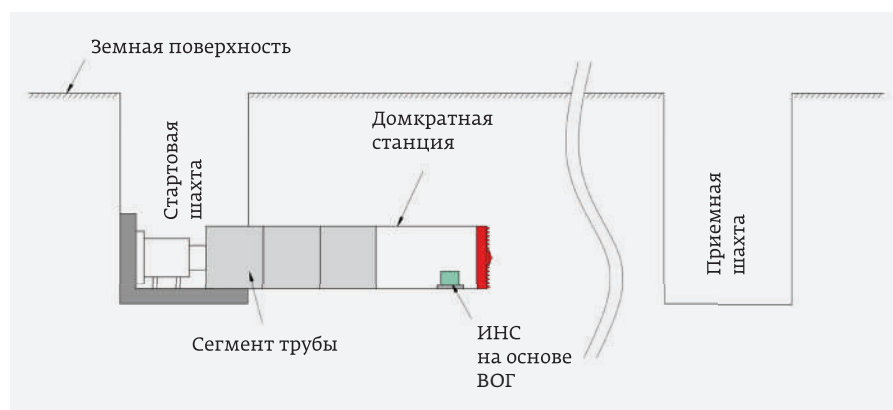
Рис. 5. Оборудование для микротоннелирования [1]
