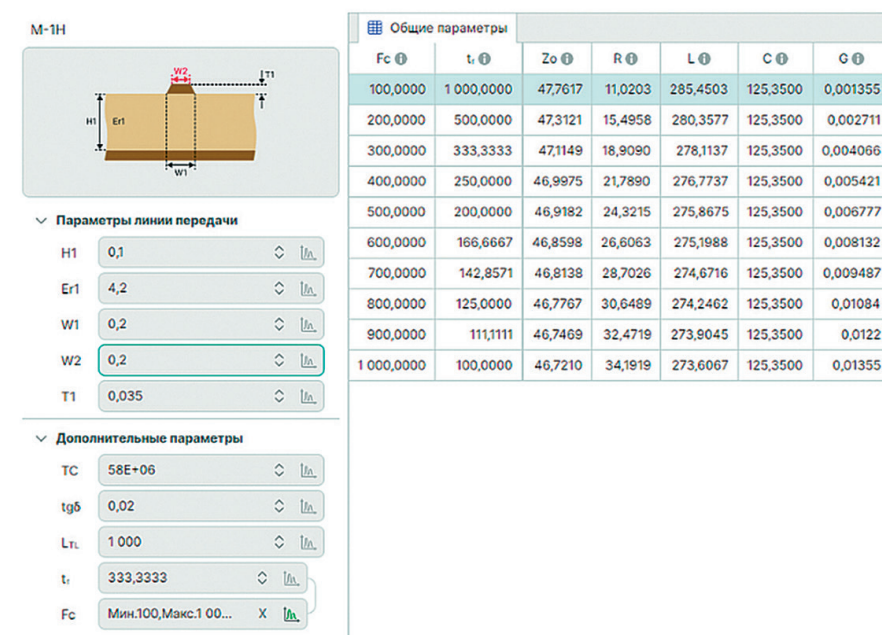
Рис. 4. Модель линии и результаты вычислений в SimPCB Lite
