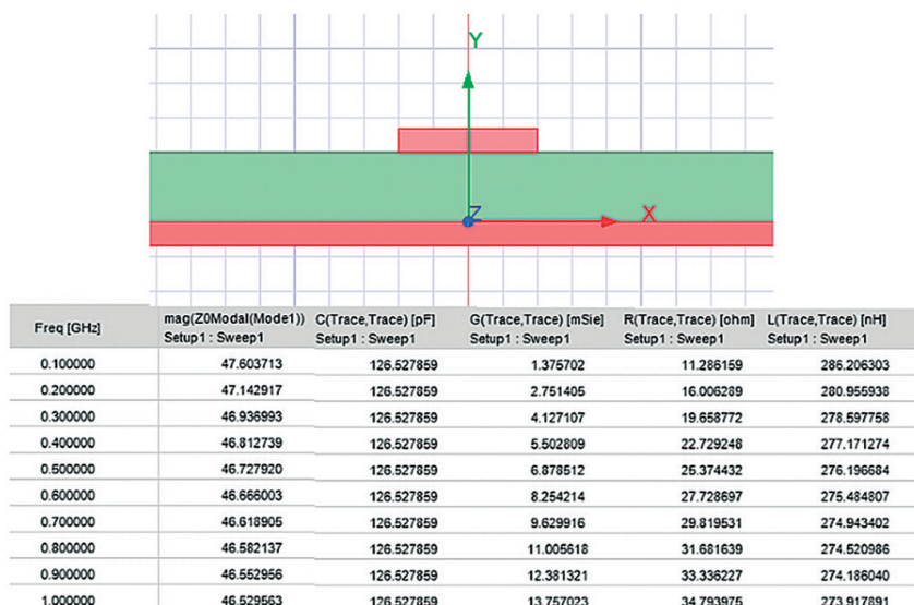
Рис. 5. Модель линии и результаты вычислений в Ansys 2D Extractor
