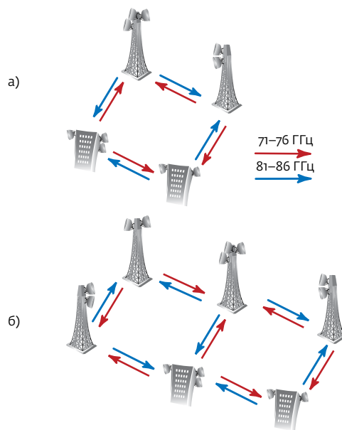
Рис.7. Сеть с кольцевой структурой (а) и со структурой из пересекающихся колец
