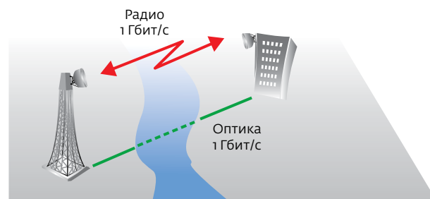
Рис.9. Применение РРЛ E-диапазона для резервирования оптического кабеля
