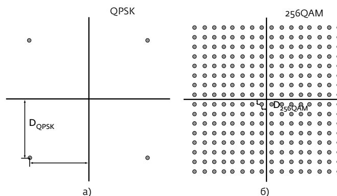
Рис.6. Увеличение межсимвольного расстояния на диаграмме Грея при использовании модуляции QPSK (а) по сравнению с модуляцией QAM-256 (б)
