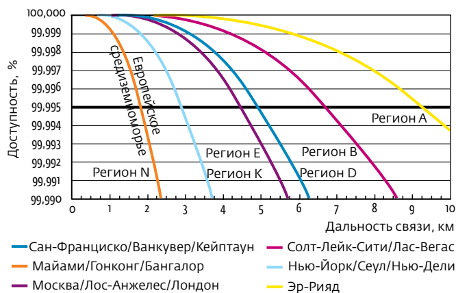
Рис.8. Зависимость между коэффициентом доступности и дальности связи для различных дождевых регионов ITU-R для аппаратуры E-Link 1000 (E-band Communications). Диаметр антенны 61 см, скорость передачи 1250 Мбит/с
