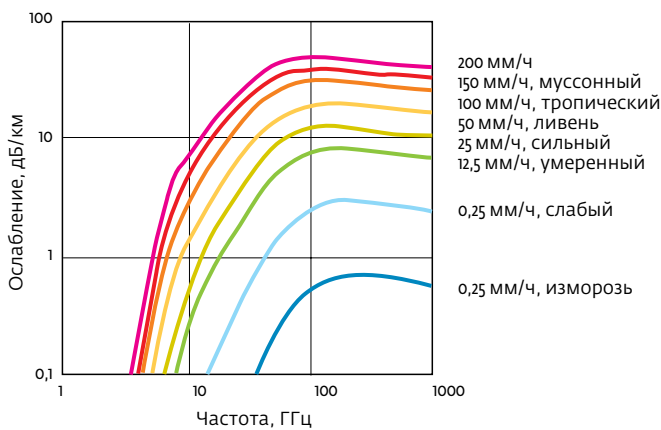
Рис.3. Затухание радиоволн, вызываемое дождем различной интенсивности
