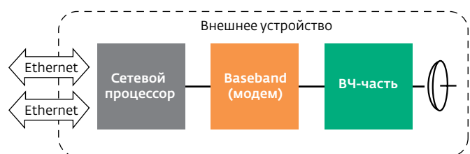
Рис.4. Общая структура трансивера Е-диапазона
