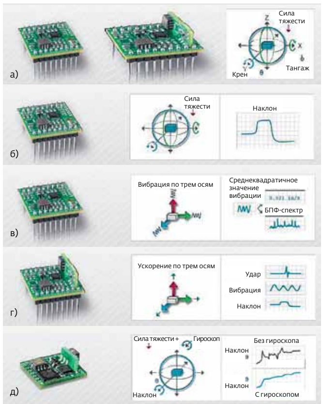
Рис. 8. Инерциальные сборки: многоосевые инклинометры SQ-SI-360DA/SQ-SI2X (а); программируемые многоосевые датчики наклона SQ-PTS (б); трехосевые датчики вибрации SQ-SVS (в), трехосевые акселерометры SQ-XLD (г); гириноклинометры SQ-GIX (д)
