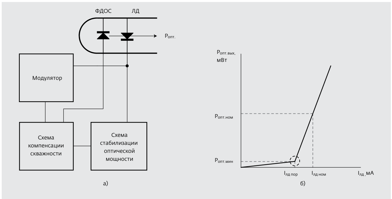
Рис.3. Функциональная схема оптического передающего устройства с компенсацией скважности входного сигнала (а) и выходная характеристика ЛД (б)
