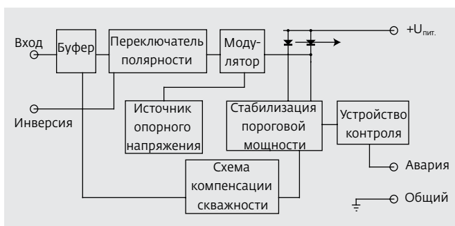
Рис.4. Функциональная схема волоконно-оптического передающего модуля OMTD-05-C-s
