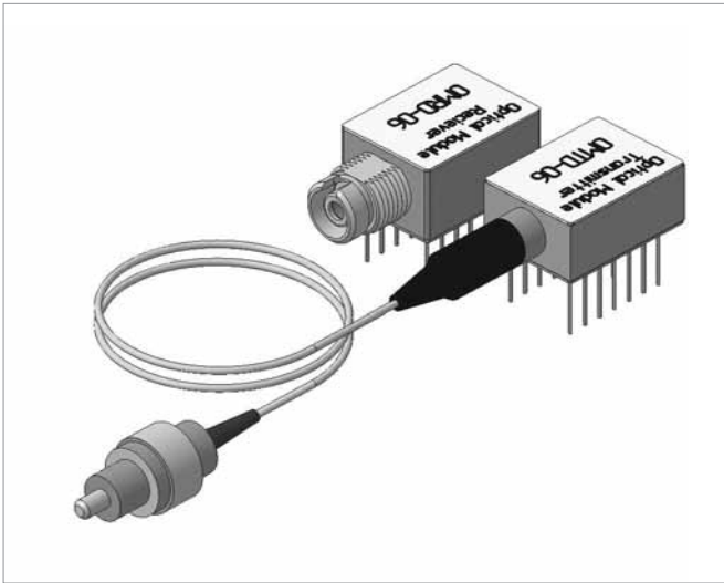
Рис. 4. Внешний вид волоконно-оптических модулей для применения в системах, использующих одномодовые (SMF) ВОЛС
