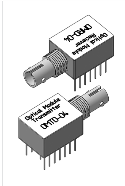
Рис. 5. Внешний вид волоконно-оптических модулей для применения в системах, использующих многомодовые (MMF) ВОЛС
