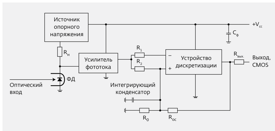
Рис.3. Функциональная схема оптического приемника OMRD-06
