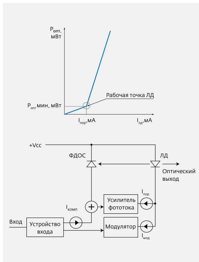
Рис.1. Положение рабочей точки ЛД на ватт-амперной характеристике и упрощенная схема компенсации скважности входного сигнала
