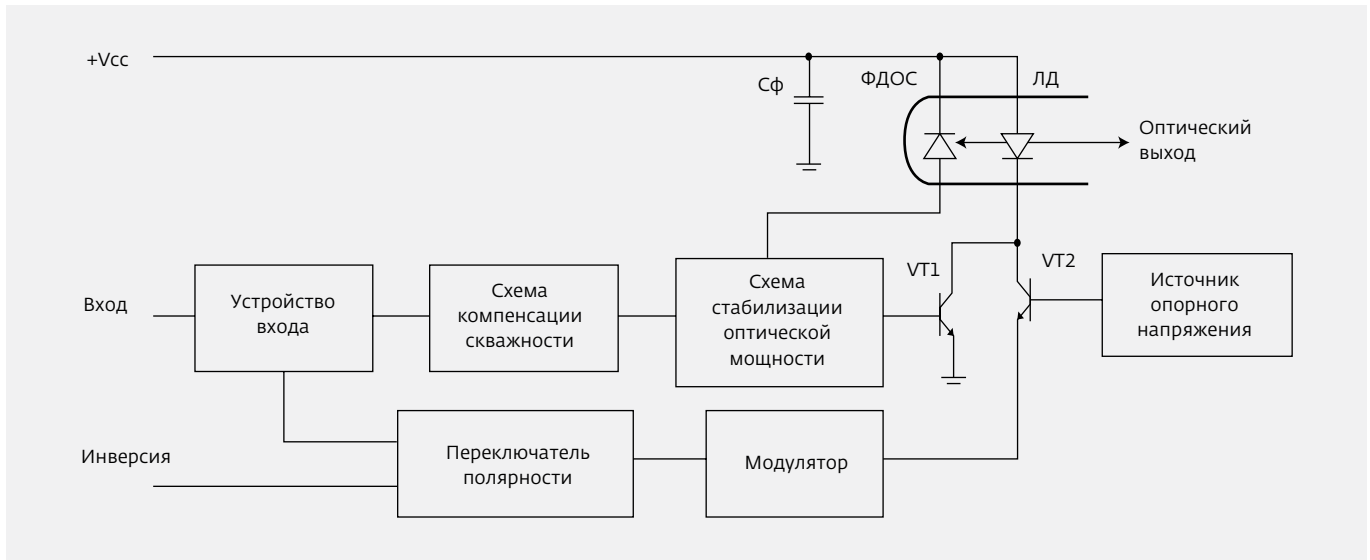
Рис.2. Функциональная схема передающего модуля, использующая ФДОС для стабилизации выходной оптической мощности
