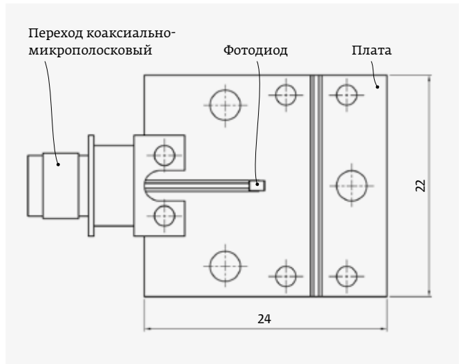
Рис. 4. Чертеж измерительной платы фотодиода
