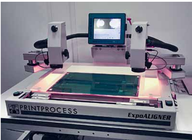
Установка автоматического оптического совмещения ExpoAligner
