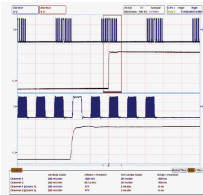
Рис. 15. Правильный выбор времени блокировки позволяет получить стабильное отображение 50-Мбит/с последовательности
