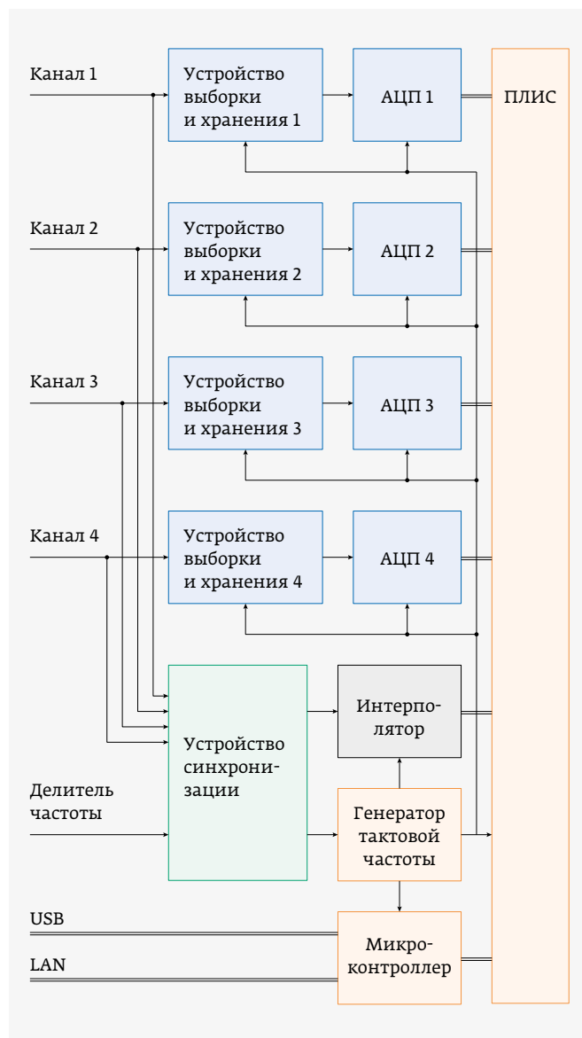
Рис. 4. Обобщенная структурная схема осциллографа АКИП-4133
