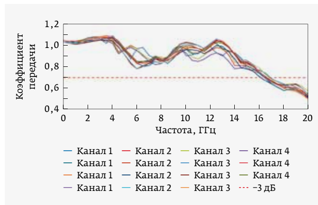
Рис. 7. Частотные характеристики, полученные при 16 измерениях в различных каналах четырех осциллографов АК ИП-4133
