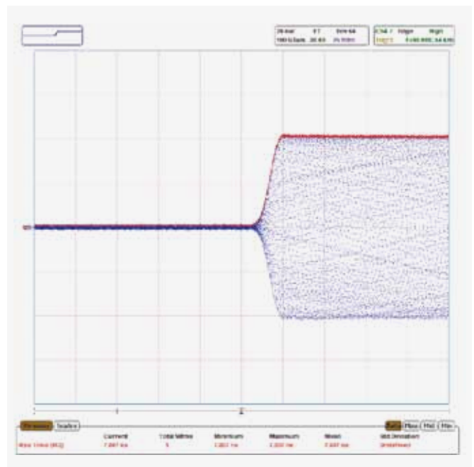
Рис. 21. Режим огибающей (красный) позволяет детектировать амплитудно-модулированный сигнал с длительностью фронта 8 нс (синий)
