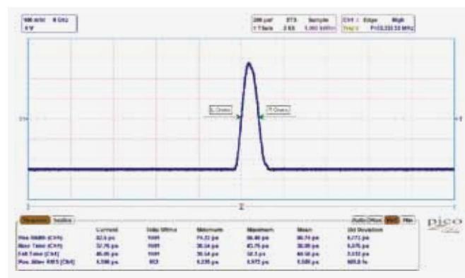
Рис. 12. Внутренняя синхронизация импульсом длительностью 81 пс
