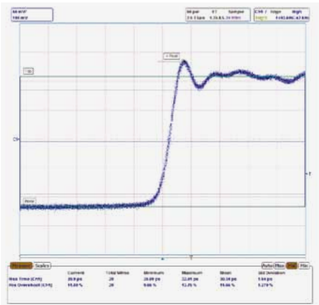
Рис. 8. Суммарная переходная характеристика осциллографа АК ИП-4133 и генератора импульсов АК ИП-3308/3 с формирователем, имеющим длительность фронта 20 пс. Суммарное время нарастания 30,31 пс
