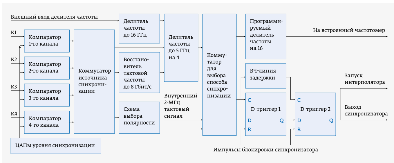
Рис. 10. Структурная схема синхронизатора
