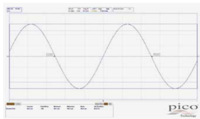
Рис. 18. Осциллограмма измерения периода усредненного 10-ГГц гармонического сигнала с погрешностью 2,2 пс
