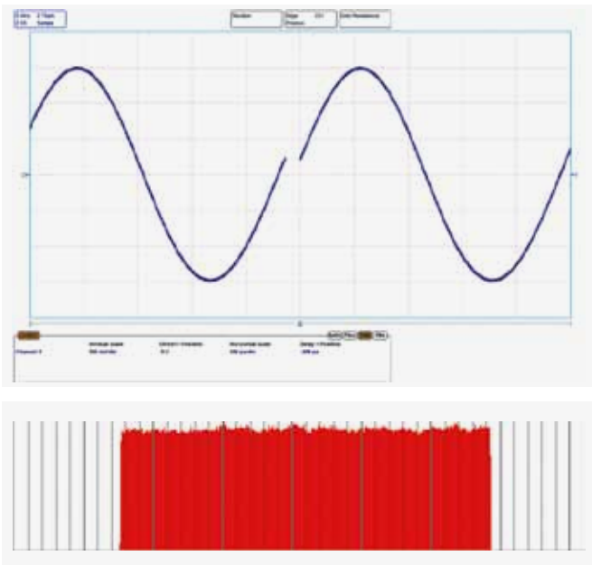
Рис. 19. Осциллограмма раскалиброванного интерполятора демонстрирует 30-пс разрыв во входном сигнале 2 ГГц. Горизонтальная шкала – 100 пс/дел. Внизу – гистограмма, используемая для калибровки интерполятора
