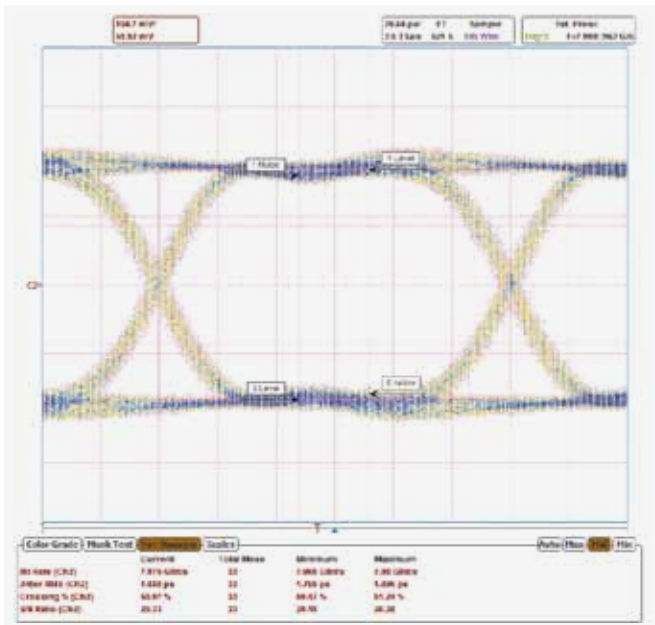
Рис. 13. Глазковая диаграмма 8-Гбит/с последовательности, зарегистрированная в режиме внутренней синхронизации с восстановлением тактовой частоты. Среднеквадратическое значение нестабильности синхронизации 1,896 пс
