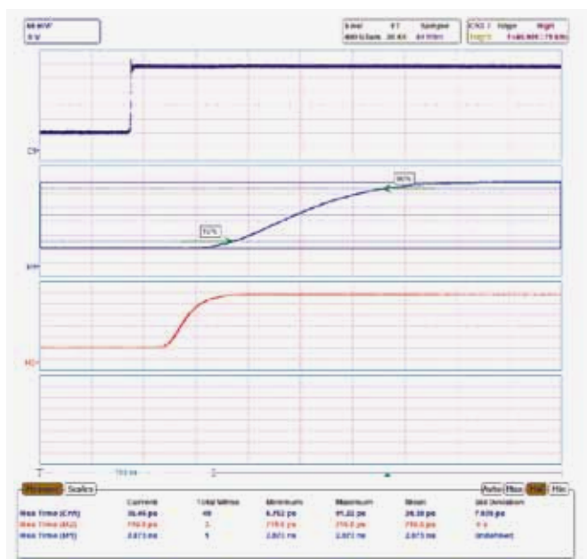
Рис. 6. Три формы переходных характеристик осциллографа АК ИП-4133 в зависимости от полосы пропускания. Сверху вниз: широкая, узкая и средняя
