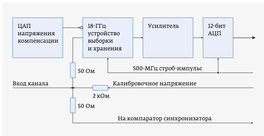
Рис. 5. Структурная схема канала вертикального отклонения
