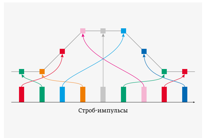
Рис. 3. Цикл захвата сигнала при случайном стробировании в эквивалентном времени
