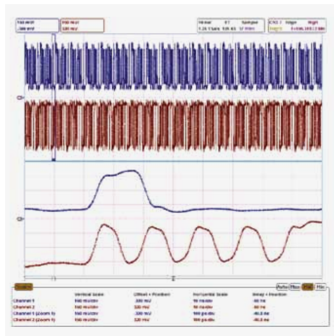
Рис. 22. Одновременное отображение двух нерастянутых и растянутых в 100 раз ПСП-сигналов
