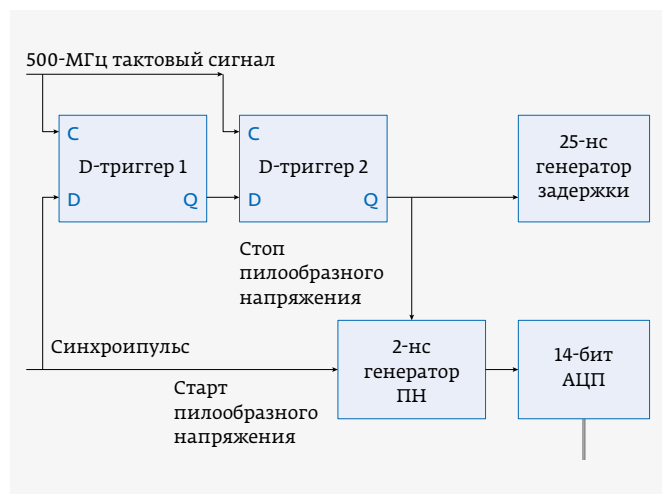
Рис. 16. Структурная схема интерполятора осциллографа АК ИП-4133
