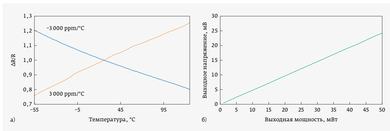
Рис. 36. Линейные зависимости R(T) РТС- и NTC-термисторов (а) и выходная характеристика термисторного измерителя мощности, представленного на рис. 35 (б)
