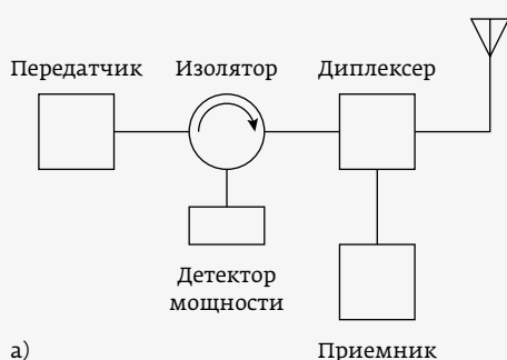
Рис. 35. Термисторный измеритель мощности: а – блок-схема тракта; б – схема измерителя
