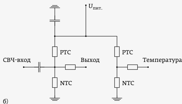
Рис. 35. Термисторный измеритель мощности: а – блок-схема тракта; б – схема измерителя
