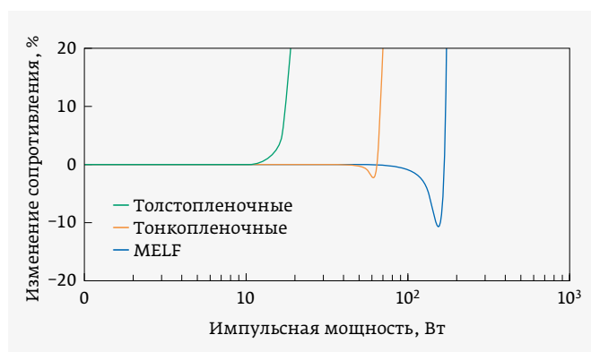
Рис. 43. Изменение сопротивления 1-кОм резисторов при импульсной нагрузке (данные компании Vishay)
