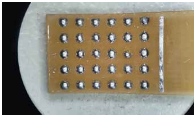
Рис. 11. Внешний вид сформированных шариков припоя на печатной плате
