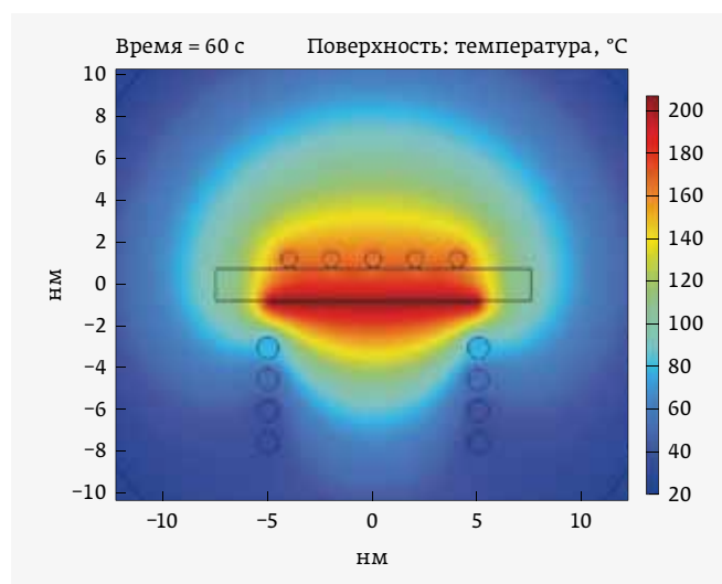
Рис. 8. Тепловые поля в зоне нагрева шариков припоя на контактных площадках печатной платы с концентратором вихревых токов
