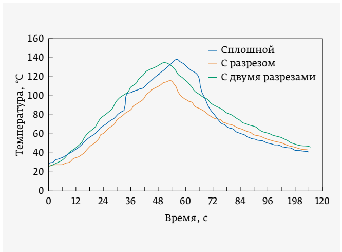
Рис. 10. Термопрофили печатной платы в процессе индукционной пайки
