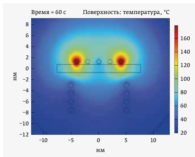
Рис. 7. Тепловые поля в зоне нагрева шариков припоя на контактных площадках печатной платы без концентратора
